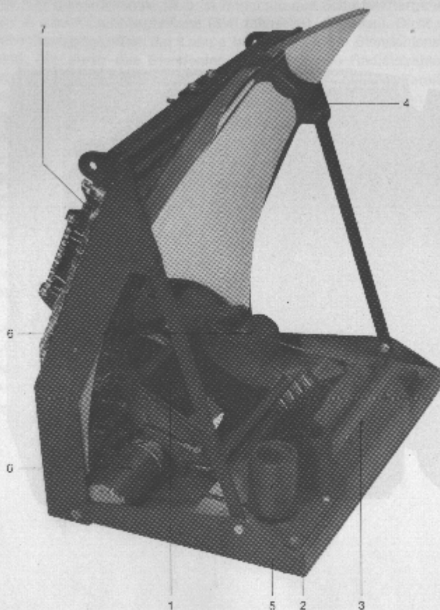
Bild 5 Scheinwerfer (Durchsichtbild)
